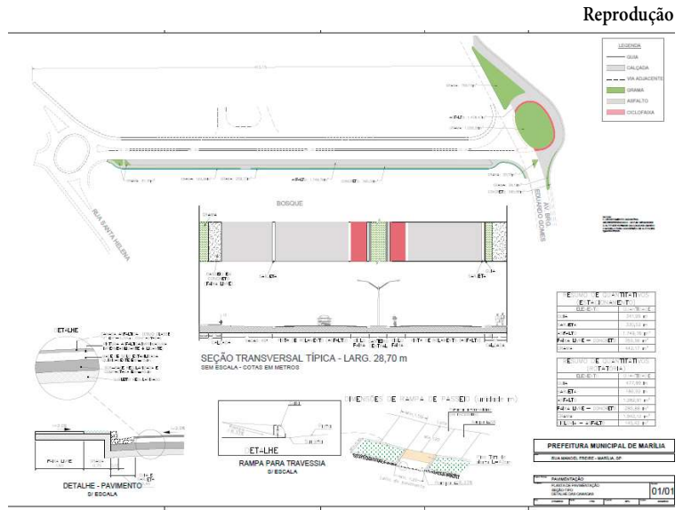
Imagem do projeto para construção de novo estacionamento anexada ao edital
