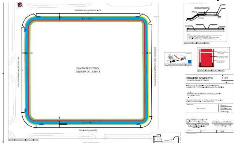
Projeto prevê a implantação de um calçamento em concreto destinado a caminhadas
